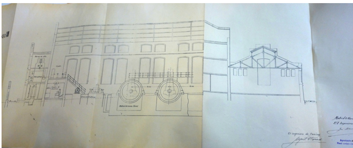
El proyecto de la Nave de Motores conservada en el AGA lleva la firma de los Otamendi en los planos, y ni rastro del arquitecto Antonio Palacios.
